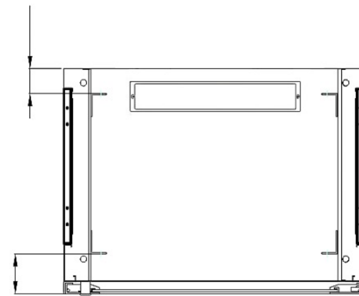
A-A Section
